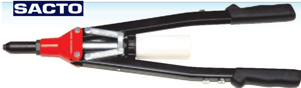
RIVDX65 Rivettatrice manuale per rivetti da \varnothing 3 \div 6,4 mm PROFESSIONALE
